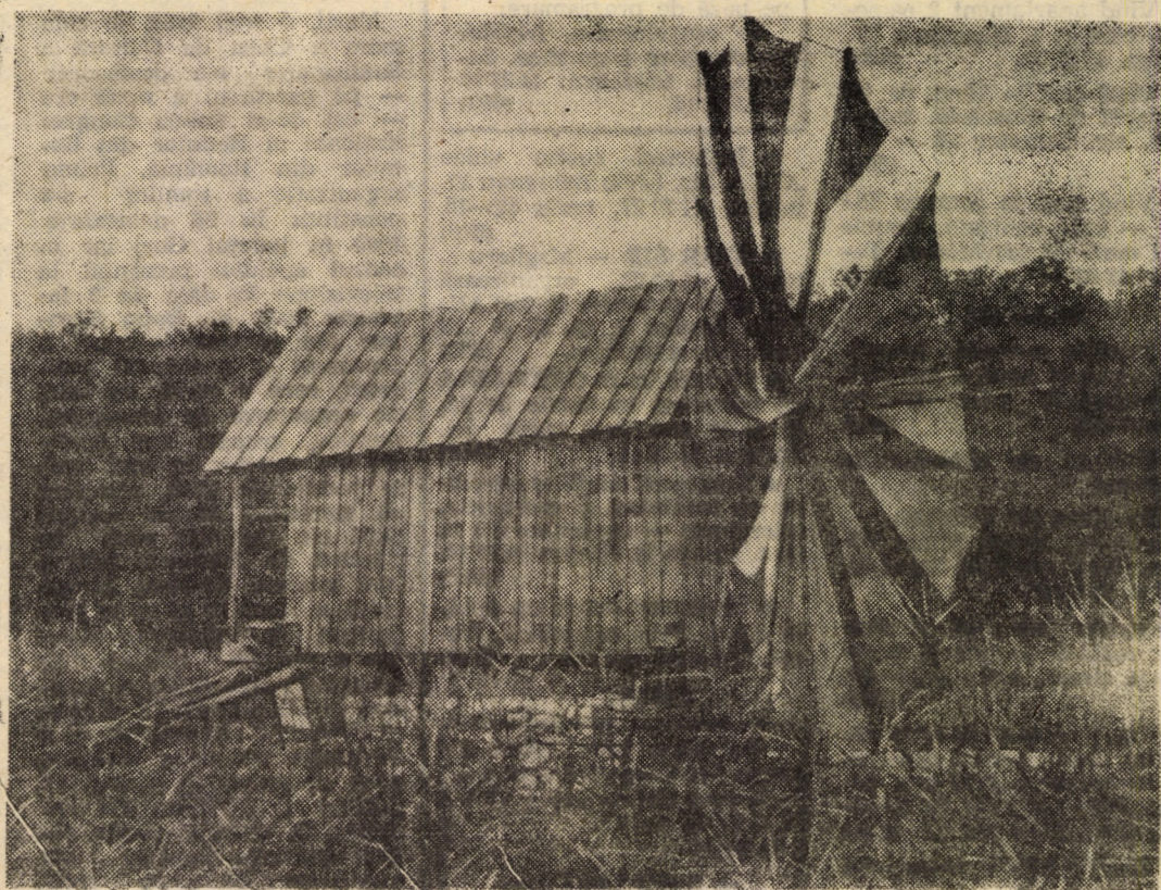
Moară de vînt cu pinze din Dobrogea.
