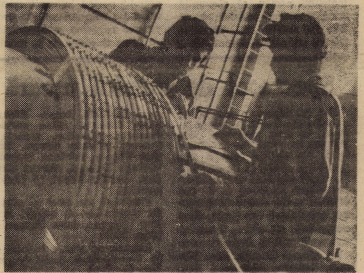
Fază de execuție a bobinajului pentru transformatoare de putere în secția reparat echipament energetic de la I.R.E. Sibiu
