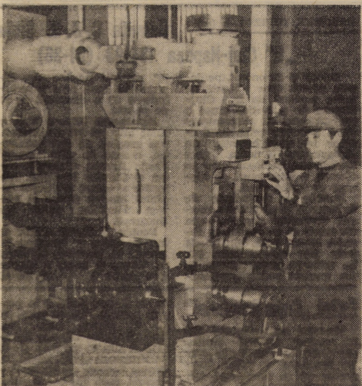
Vedere parțială a noului laminor de sîrmă pentru dinți spete, realizat nu demult în atelierul de autoutilare al Întreprinderii „Flamura Roșie” Sibiu Foto: Fred NUSS
