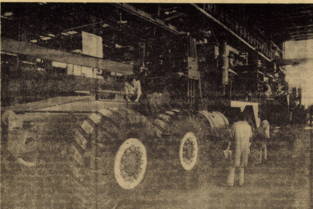
În imagine: autoremorcherul de mare tonaj destinat transportului de utilaj petrolier, aflat în faza de montaj final la Întreprinderea mecanică Mirșa — unitate recent vizitată de secretarul general al partidului, tovarășul NICOLAE CEAUȘESCU Foto: Fred NUSS
