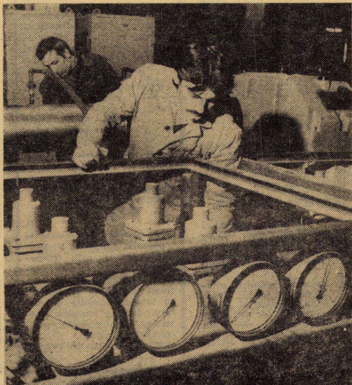
Întreprinderea mecanică Sibiu: lăcătușii Liviu Tănase și Ioan Cojocar u efectuind probe tehnologice la un extrudor pentru cauciuc cu alimentare la rece, tip ECR 120, al cărui beneficiar va fi Centrala industriei de prelucrare mase plastice și cauciuc. Prin realizarea acestui utilaj, colectivul întreprinderii contribuie la reducerea unor importuri. Foto: Fred NUSS
