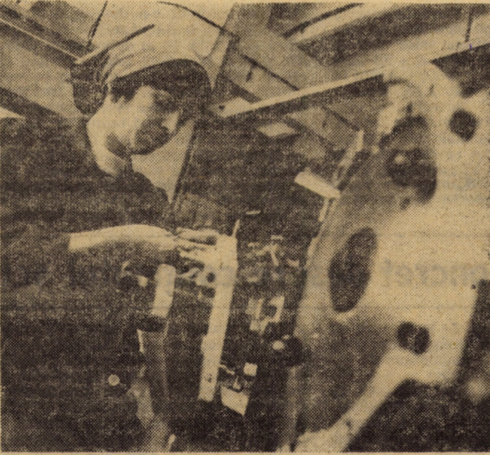
Recent, în secția metal II, ace textile, a întreprinderii „Flamura roșie“ Sibiu, a fost dată în funcțiune o mașină de scurtat, marcat și îndreptat ace pentru mașini de cusut, realizată în cadrul atelierului de autoutilare al întreprinderii. Efectuînd trei operații consecutive, noul utilaj asigură o creștere substanțială a productivității muncii. Foto: Fred NUSS
