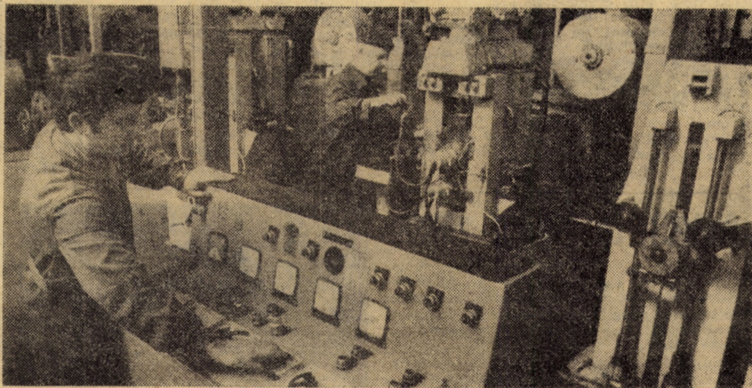
Întreprinderea „Flamura roșie” Sibiu. Instalația automată de laminat sirmă din secția metal II, deservită într-unul din schimburi de Cornel Burnete, șef echipă, și muncitorul Gheorghe Tudorică
