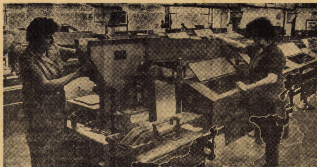
Recent, la I.P.L. Sibiu, sector creioane, au fost puse în funcțiune o serie de noi utilaje și linii tehnologice moderne. În imagine: liniile automate de vopsit creioane Foto: Fred NUSS
