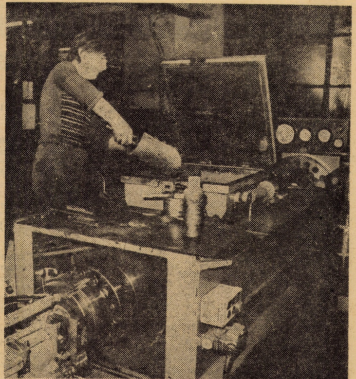
I.P.L. Sibiu. Agregatul din imagine asigură minele pentru secția de fabricarea creioanelor, utilaj de înaltă complexitate și mare capacitate Foto: Fred NUSS
