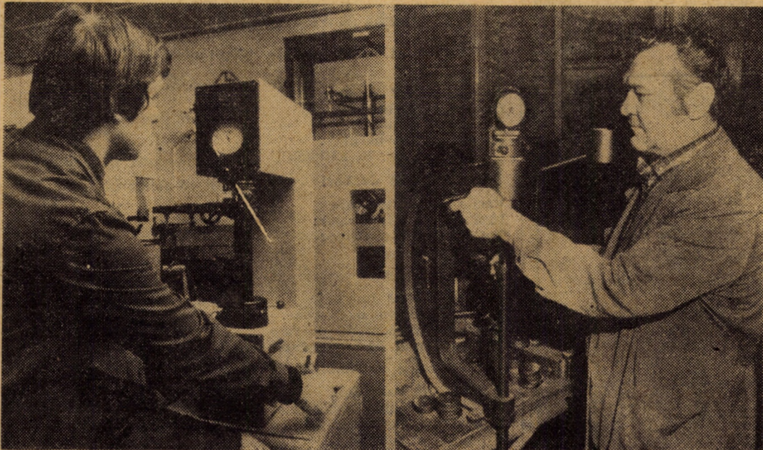
Azi, vă prezentăm două dintre noile produse realizate la întreprinderea „Balanța” Sibiu: aparatele tip „Rockwell” cu ceas comparator și cu cuplaj de repoziționare (stînga) și „Rockwell” portabil (dreapta). Foto: Fred NUSS
