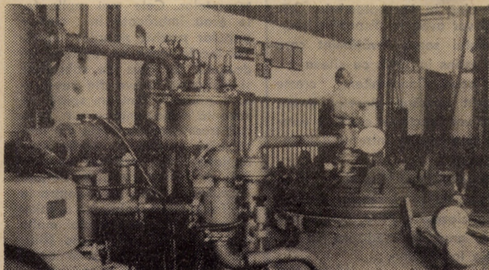
Cu ajutorul unei instalații complexe de recept sîrmă în cuptoare speciale cu atmosferă controlată, la sectorul metal II al întreprinderii „Flamura roșie” Sibiu se obține o îmbunătățire substanțială a calității sîrmelor, necesare producției de accesorii textile, realizate azi într-o mare varietate de tipodimensiuni Foto: Fred NUSS
