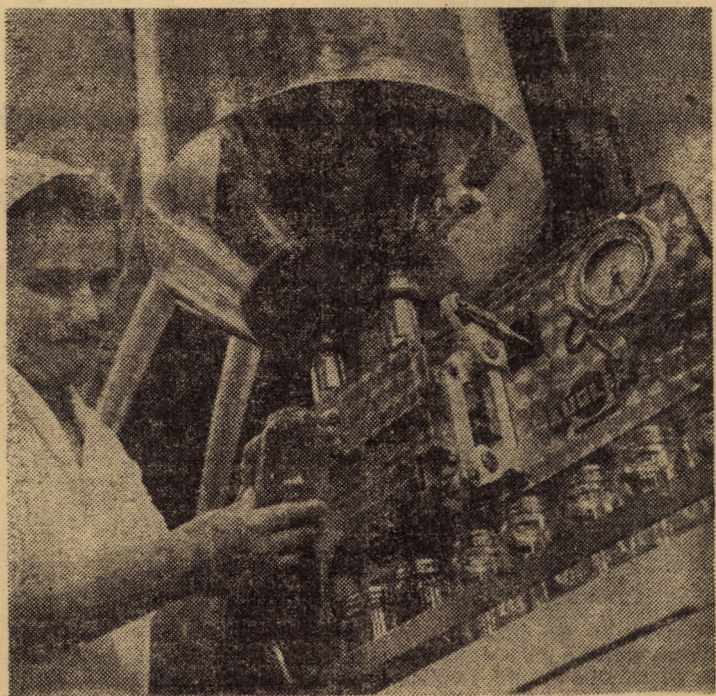
La Întreprinderea de omogenizarea mierii și producție alimentară Sibiu, utilaje moderne asigură concomitent îmbutelierea, etichetarea și căpăciul borcanelor cu miere.
