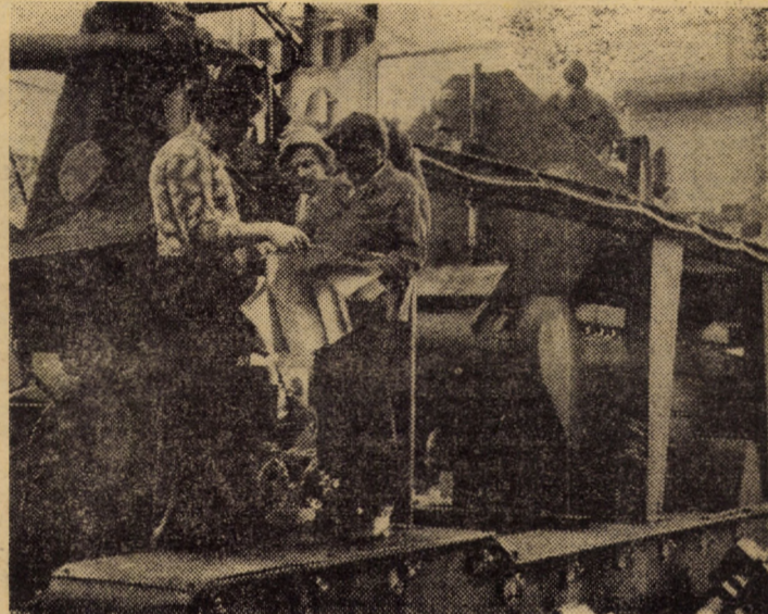
O realizare în premieră în cadrul secției mecanică II a întreprinderii „Independența” Sibiu: mașina de format destinată industriei metalurgice, aflată în stadiul de montaj final. Foto: FR. NUSS
