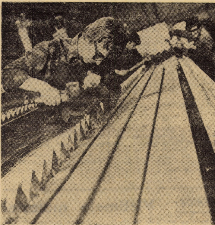
Utecistul Emilian Scirneciu, lăcătuș în atelierul de montaj al întreprinderii „Independența” Sibiu lucrînd la finisarea grebelor pentru grătarul mobil la paturile de răcire ale laminoarelor
