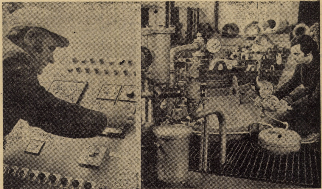
Secția metal II, a întreprinderii „Flamura roșie” Sibiu: Linia modernă pentru recoacerea în vid a sirmelor necesare accesoriilor textile Foto: FRED NUSS
