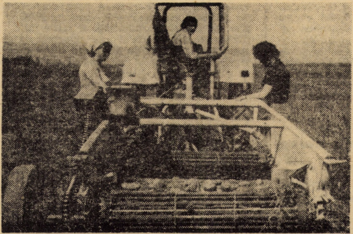
Secvență de la recoltatul cartofilor cu M.S.C.-1 pe terenurile Cooperativei agricole de producție din Cirta
