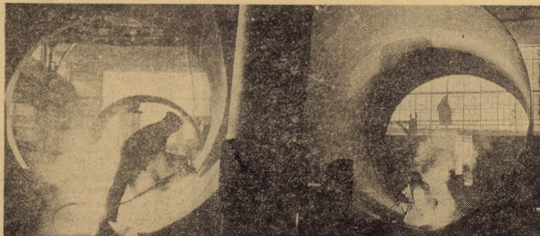
Peisaj industrial sibian 1978: sudarea și finisarea tronsoanelor de mari dimensiuni la cazangeria „Independența” Sibiu Foto: FRED NUSS
