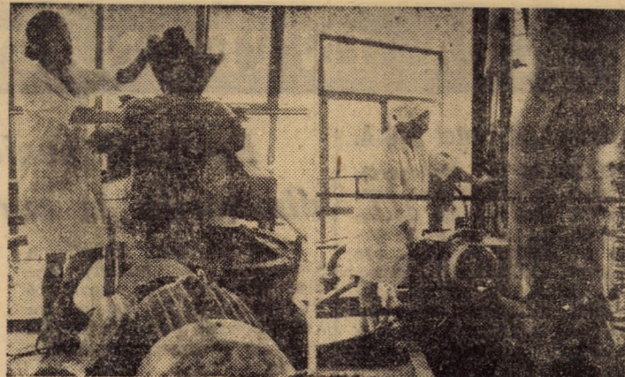
Noi capacități de producție recent intrate în funcțiune la întreprinderea de bere și amidon Sibiu: stînga: moară pentru măcinat hamei dreapta: cazan pentru filtrarea mustului de bere
