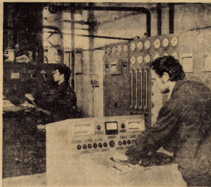
Conducerea și urmărirea tuturor utilajelor din fluxul de fabricație a întreprinderii pentru producerea nutreturilor combinate Sibiu se efectuează cu ajutorul schemei sinoptice instalată în camera de comandă centralizată Foto: FRED NUSS
