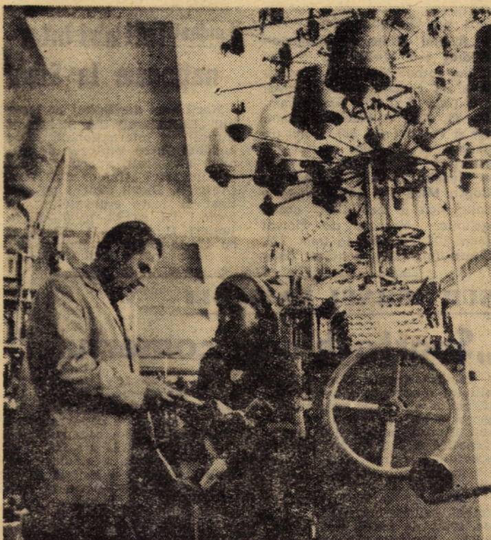
Întreprinderea de ciorapi și mănuși, Agnita. Prin introducerea în ciclul de producție a noilor mașini circulare automate de tricatat mănuși cu contexturi jacquard — utilaje realizate prin autoutilare — eficiența economică se ridică anual la 350 000 lei
