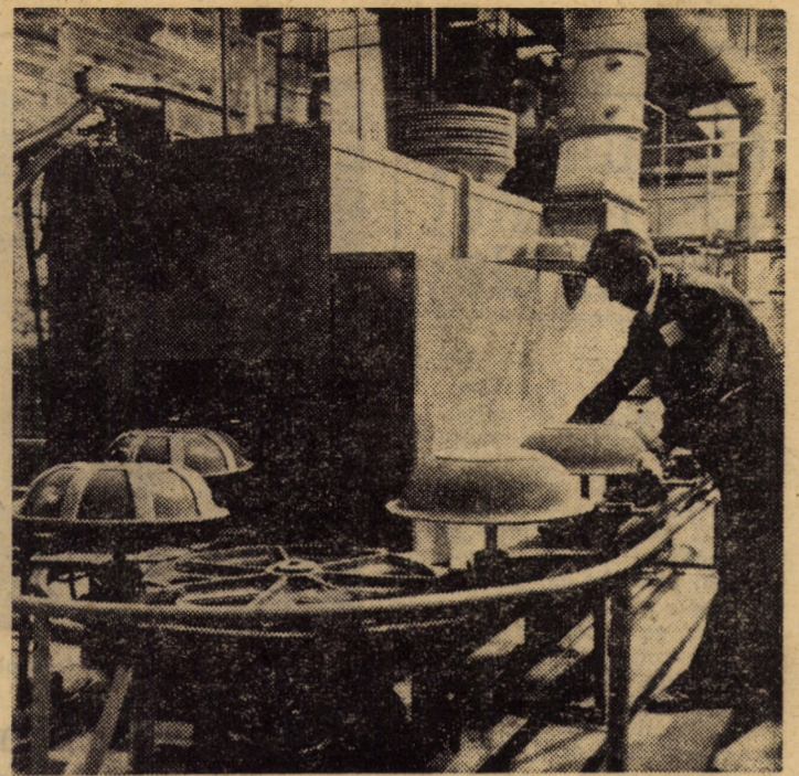
„Emailul roșu” Mediaș: una din cele două mașini de emailat realizate prin autodotare și aflate în prezent în probe tehnologice. Cu aceste două noi utilaje s-a obținut o linie tehnologică în flux continuu pentru emailarea vaselor mari. Foto: FRED NUSS
