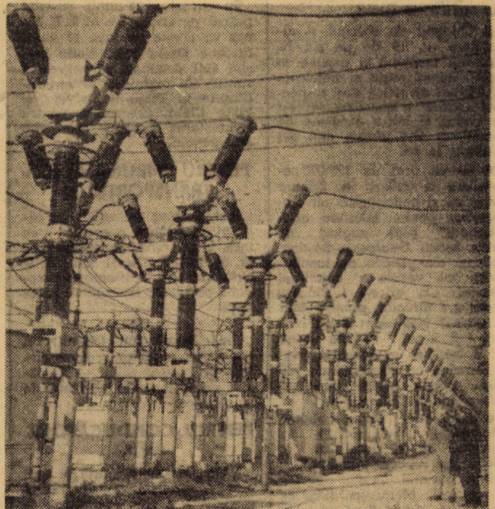
O adevărată „pădure” de conductori electrici purtînd spre beneficiarii energia necesară industriei. În foto: stația de 220 KV Sibiu-sud
