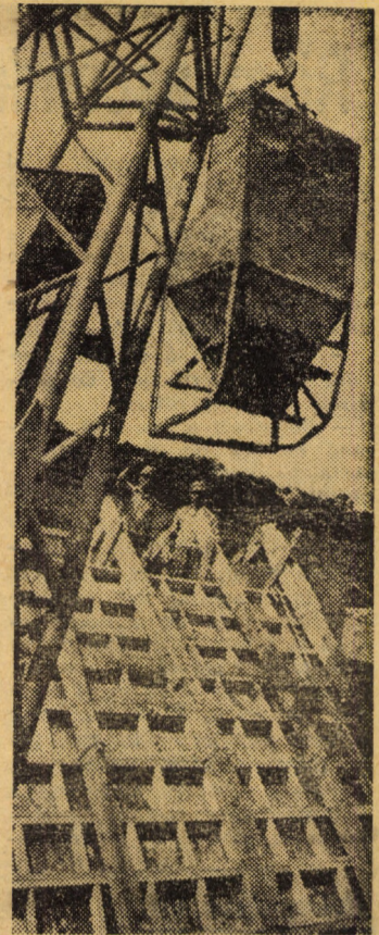
Șantierul de la Ighis Nou. Lucrări la conducta de aducțiune a barajului Copșa Mică
