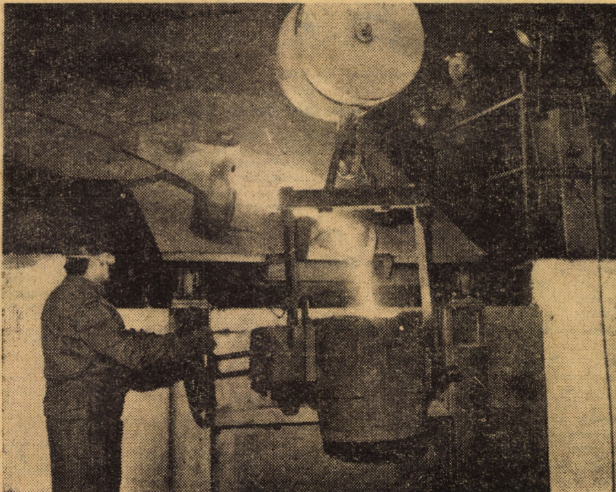
Cuptor electric pentru topirea oțelului, fabricat de întreprinderea „Îndeapănța” Sibiu
