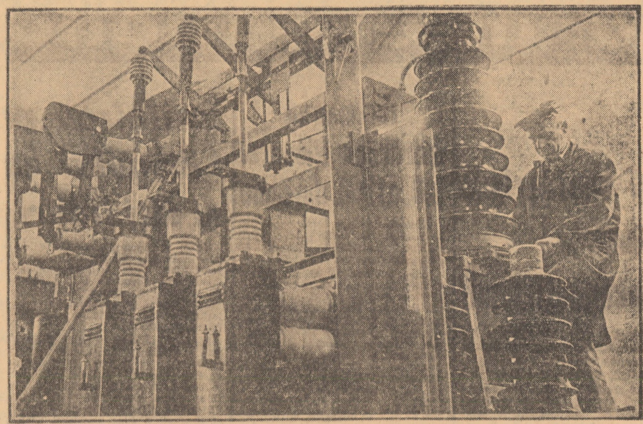
Sectorul de reparat Interupătoare de înaltă tensiune de la I.R.E. Sibiu, condus de Grigore Moldovan, șef de echipă. În fotografia de față — montînd un izolator
