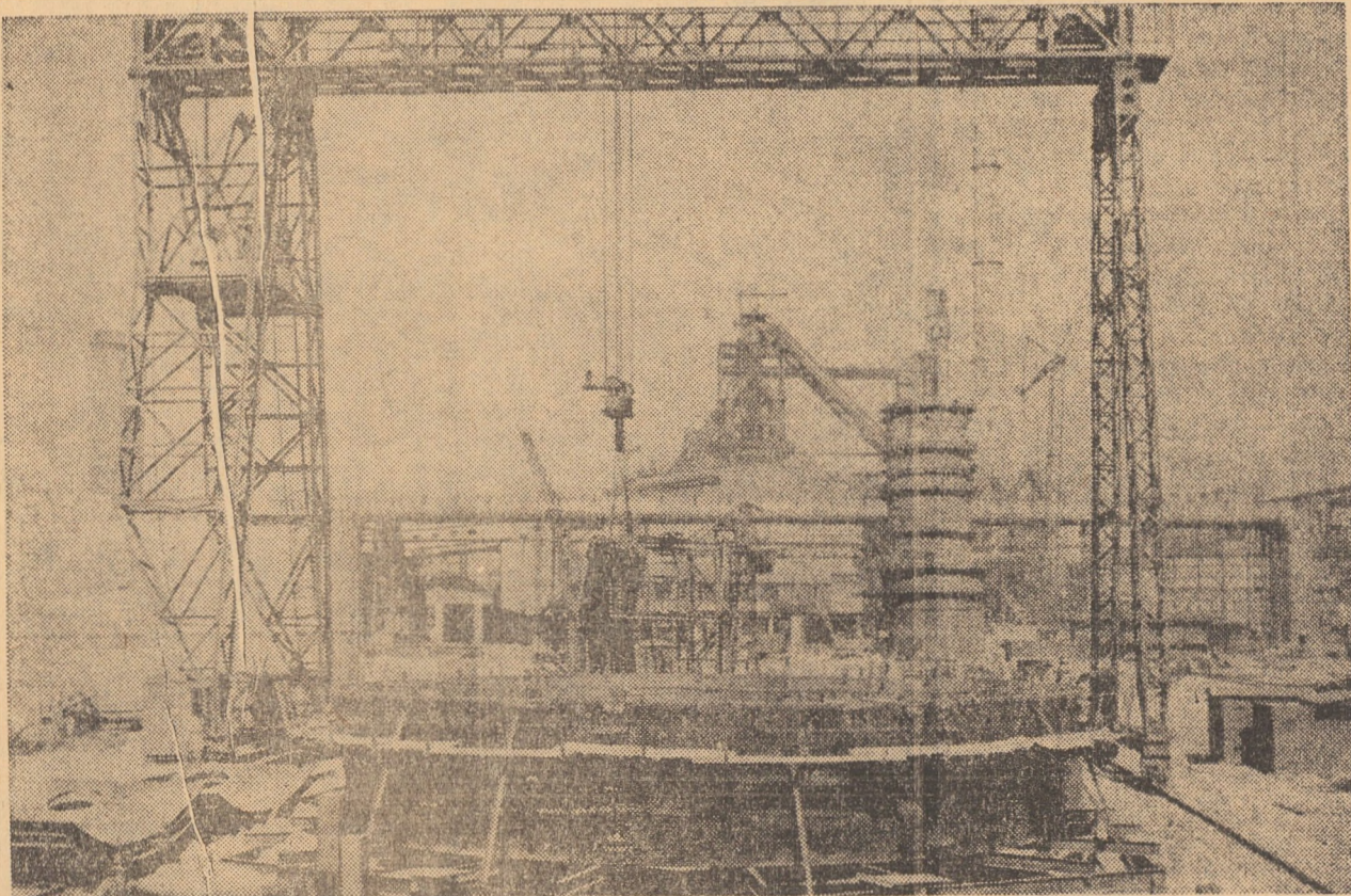
U.R.S.S. METALUL — BAZA INDUSTRIEI SOVIETICE. La uzina metalică din Ovolpejk se construiește cel mai mare furnal din țară cu o capacitate de 3200 mc, care va elabora 2,3 milioane tone fontă pe an. Acest furnal este unul din cele 6 mari furnale, care vor fi construite în acest cîcinal. În perspectivă se prevede construirea de furnale cu o capacitate de 5000 metri cubi. În foto: se montează mantaua furnalului
