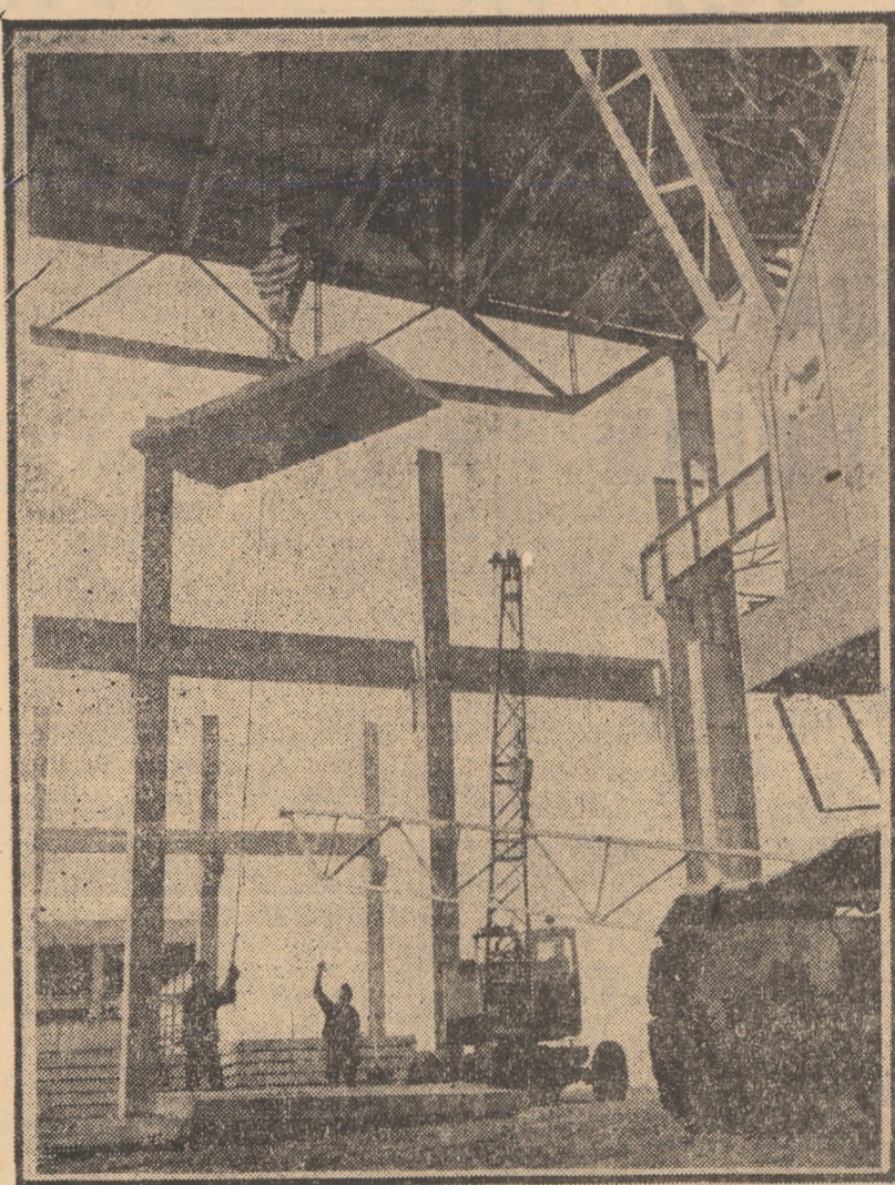
Montarea chesoanelor la noua hală de turnătorie a uzinei „Independența” II Sibiu, pe șantierele de construcții
