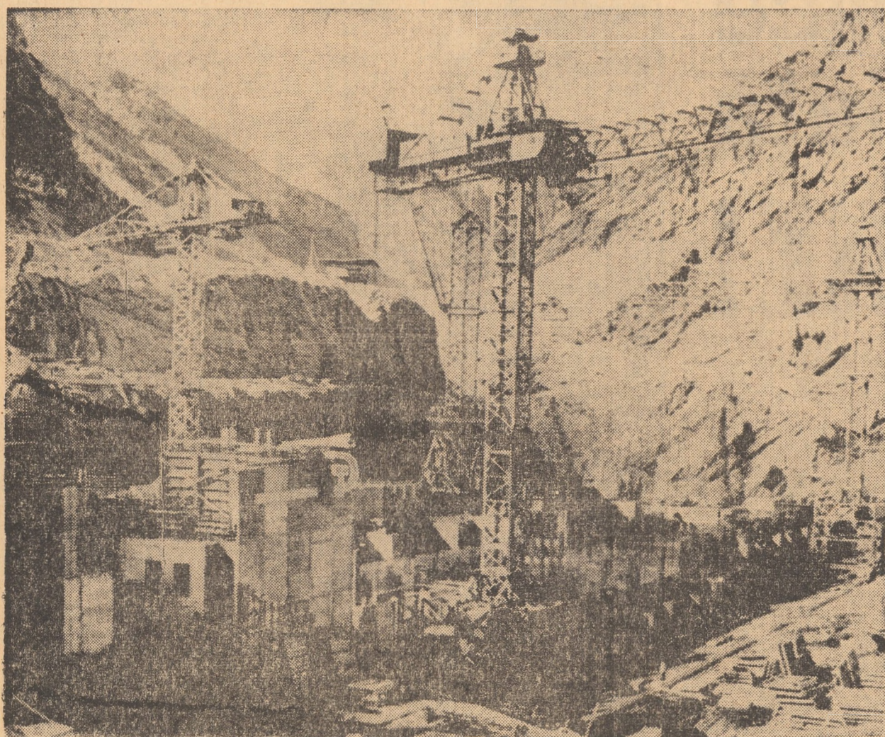
U.R.S.S. Pe șantiierul hidrocentralei Nurek din Tadzhikistan
