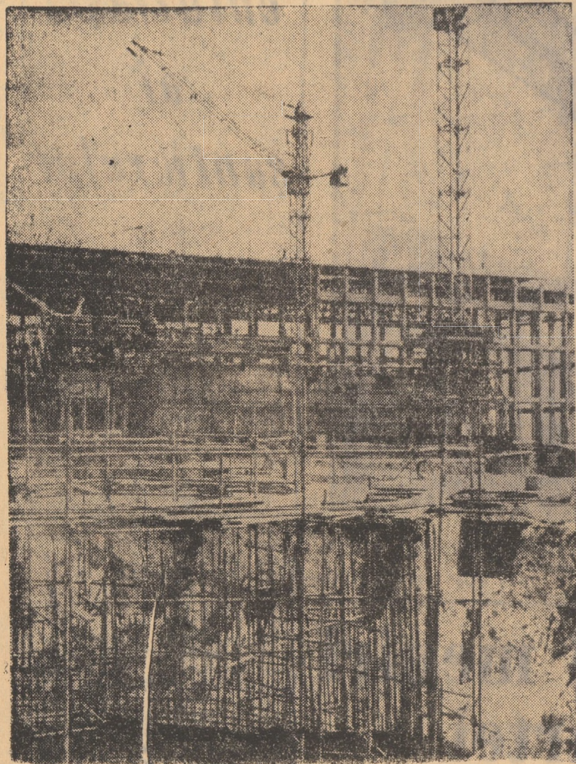
R.P. BULGARIA. Îngă orașul Kozlodou, districtul Vratza se află în construcție prima stație atomică din Bulgaria. Construcția ei se va desfășura în două etape: prima parte va fi terminată în 1975, va avea 440 megawați producând anual 5-6 miliarde kWh energie electrică. A doua parte va fi terminată în anul 1978. În foto: vedere generală a stației atomice
