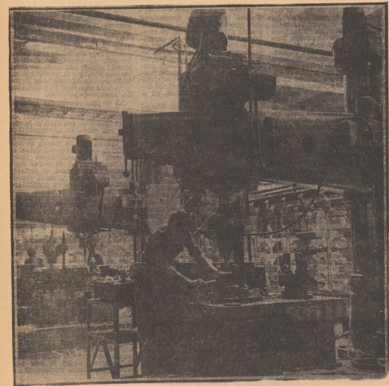
Printre angajamentele luate de muncitorii de la U.P.A.S. în cinstea zilei de 23 August a.c., harnicul colectiv de muncitori şi tehnicieni al atelierului cardane şi mecanisme de direcţie, şi-a propus depăşirea planului cu aproape 600.000 lei. În fotografie: grupul de maşini de găurit de mare productivitate
