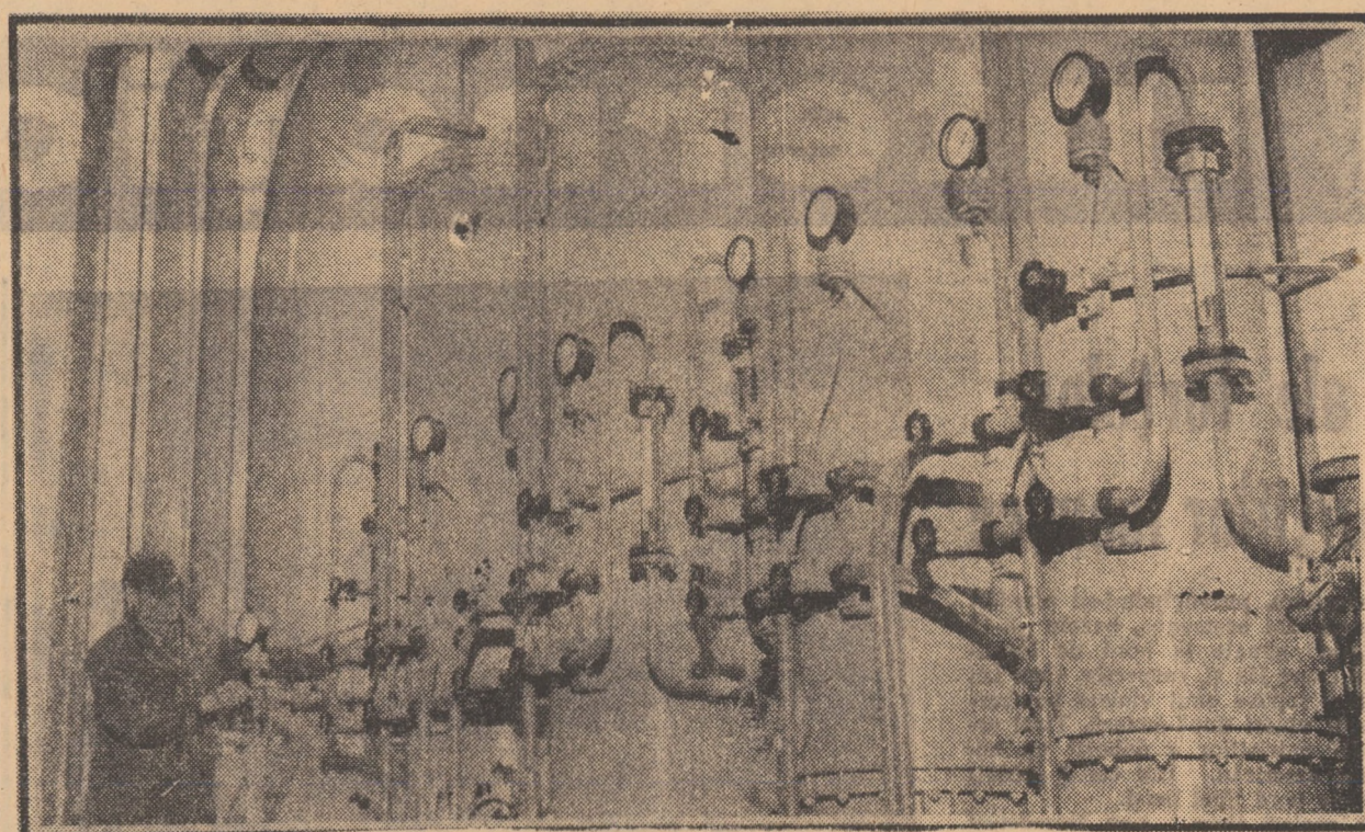
Instalații moderne de dedurizare a apei la uzina Emailor roșu Mediaș
