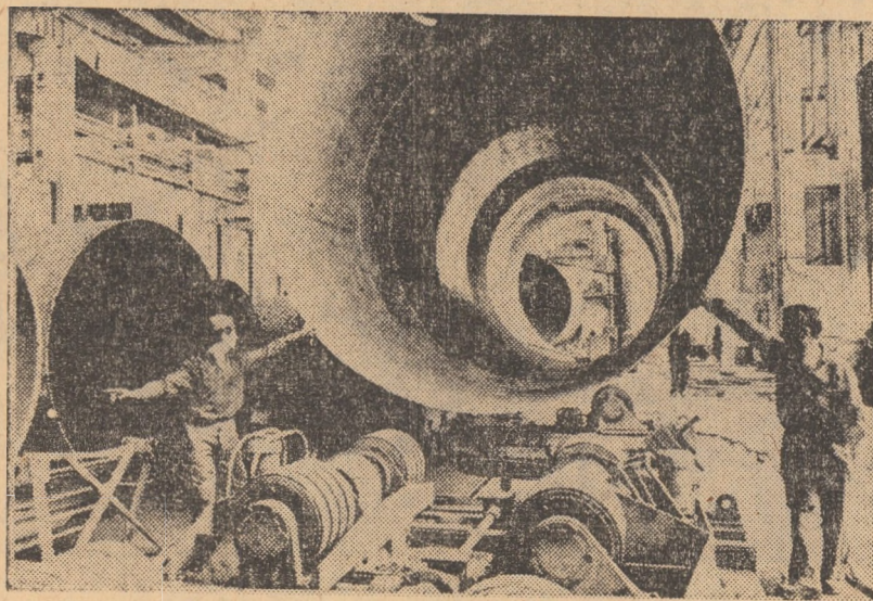
REPUBLICA DEMOCRATĂ GERMANĂ. Aspect din hala de asamblare pentru containere mari de la uzinele chimice „Germania” din Karl-Marx Stadt
