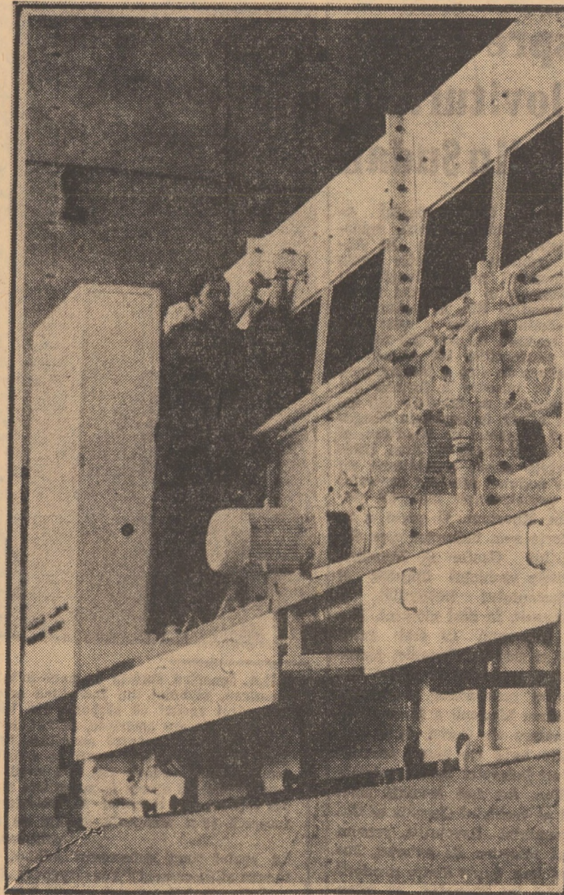
Recent, fabrica „Berea Sibiului” a fost dotată cu un utilaj modern de spălat sticle care se află în curs de montare. Noua mașină are o capacitate de 16.000 sticle/oră.
