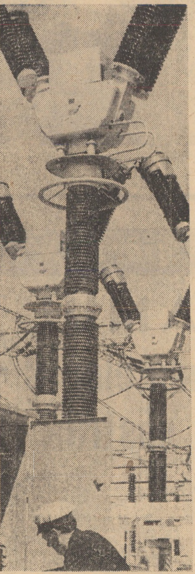
În cinstea zilei de 23 August, colectivul de muncă de la „Electromontaj” Sibiu, muncește cu avânt pentru realizarea înainte de termen a stațiilor și a rețelelor care contribuie la creșterea potențialului energetic național. În clișeu: lucrările la o nouă stație sunt încheiate
