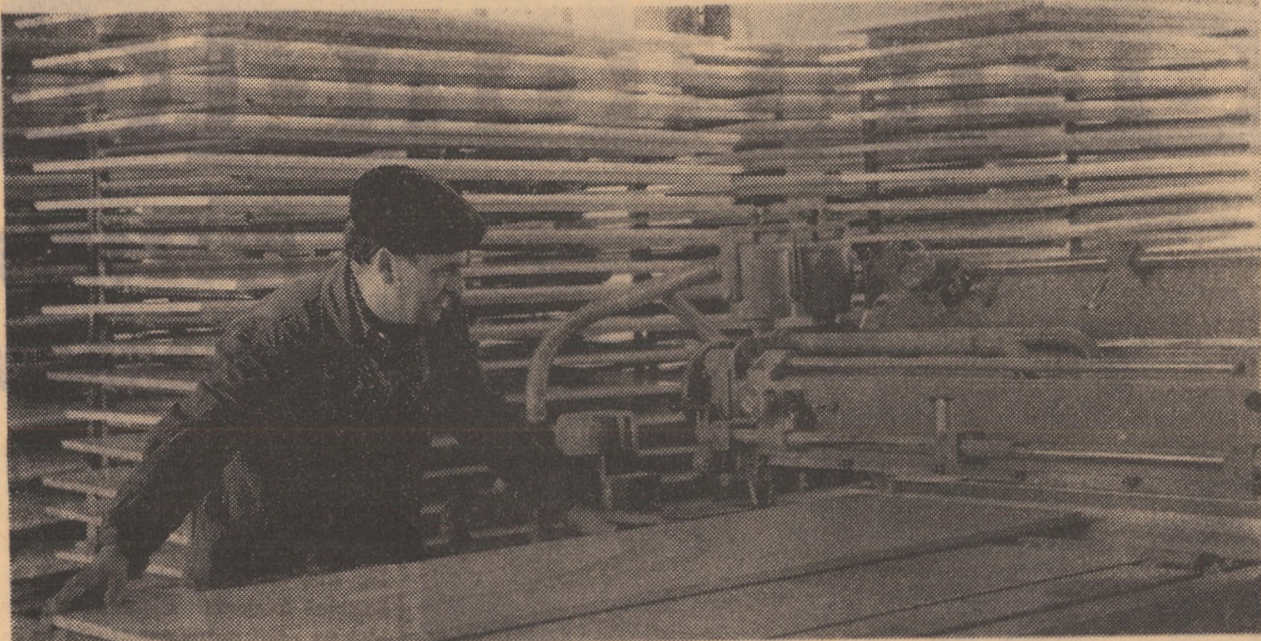
La profil „Republica” din Sibiu, la secția a II-a mobilă, a intrat de curând în funcție o nouă mașină de turnat lacuri carboamidice, folosite la finisarea mobiliei. Noul utilaj lucrează alternativ cu două capete de turnare, realizând, într-un schimb, un număr de 1 000 panouri finisate
