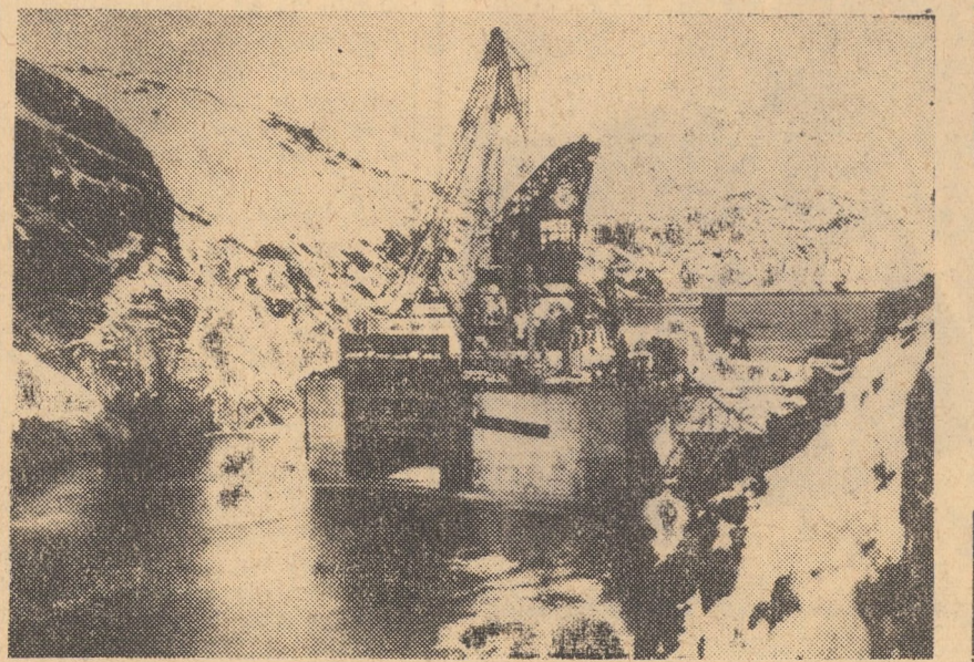
U.R.S.S. — În regiunea Murmansk, în estuarul Kistol al Mării Albe a început în ajunul anului trecut construcția primei centrale electrice experimentale pe bază de flux și reflux. În cursul anului această centrală a început să dea curent. Puterea acestei centrale nu este mare, dar mare este importanța sa pentru proiectarea viitoarelor centrale electrice pe malul mării Barent și pe cel al Mării Albe. — Prima centrală electrică pe bază de flux și reflux, în estuarul Kistol
