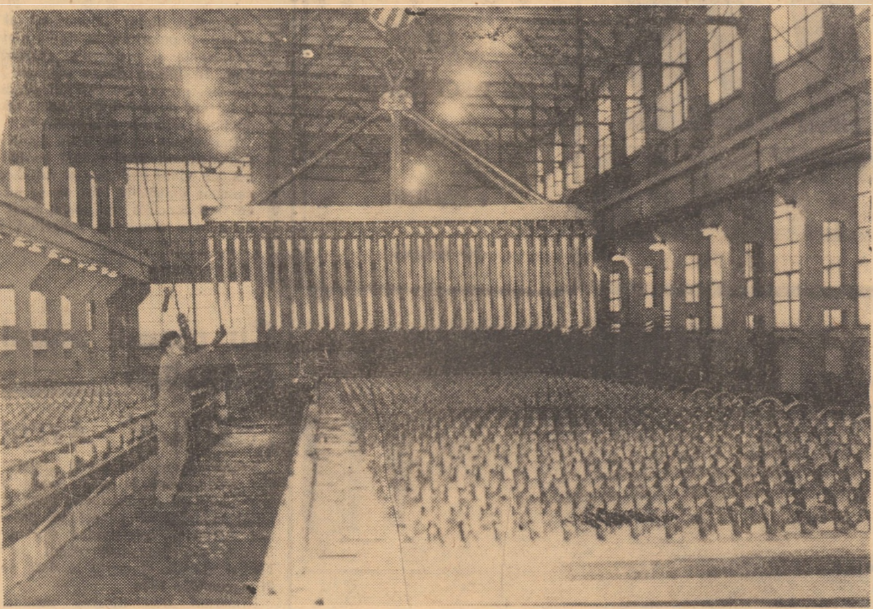
În această hală imensă, printre cioturi de plumb alinate într-o ordine perfectă, un om dirijează prin telecomandă un alt "cîrd" de bare grele în noua instalație electrolitică a plumbului de la U.C.M. Copșa Mică.
