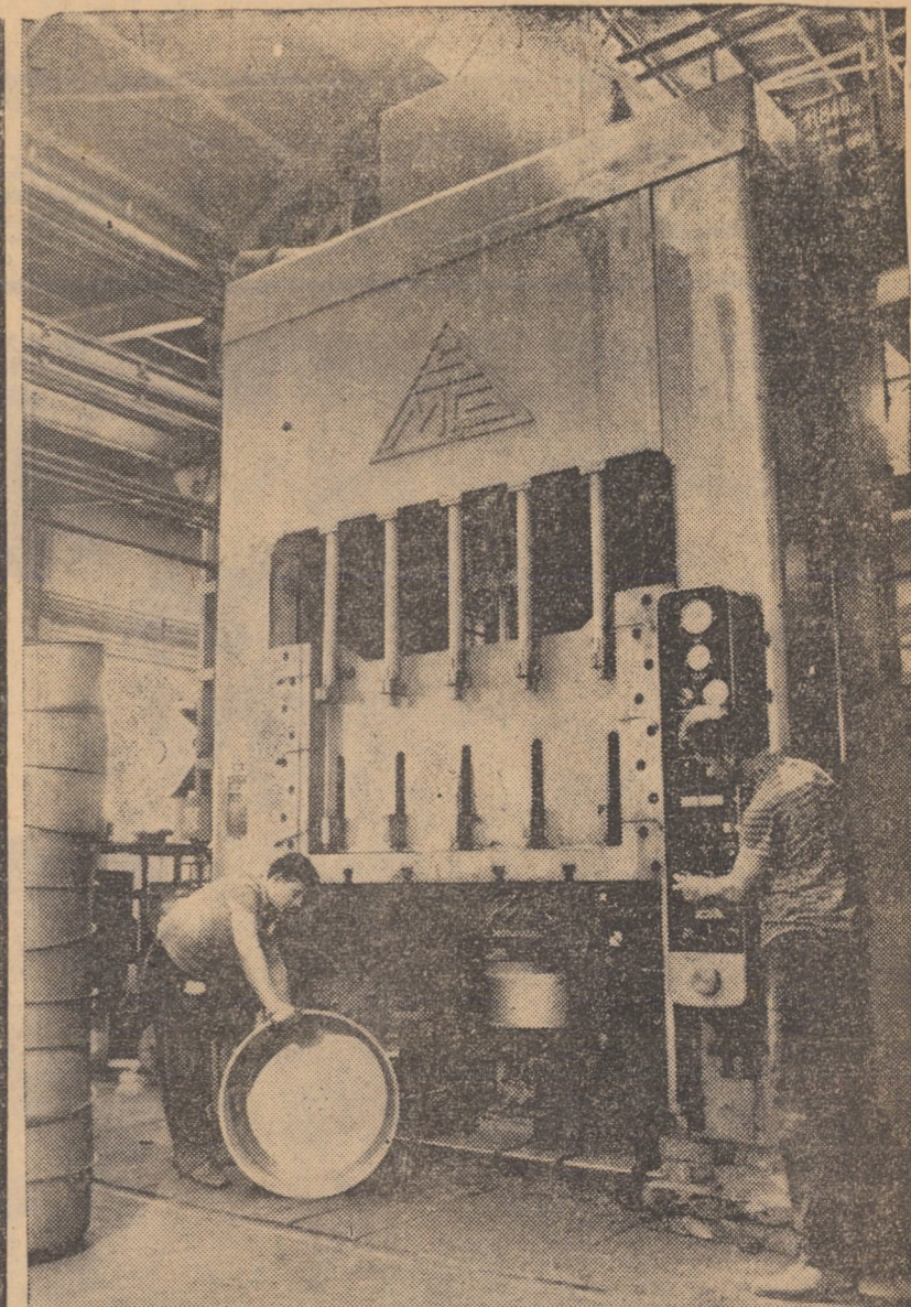
Operația de ambutisare a cuvelor pentru betoniere, produse de uzina „Independența” din Sibiu, se efectuează cu ajutorul prese hidraulice de 600 tone, utilaj cu o productivitate de peste 300 cuve în 8 ore.
