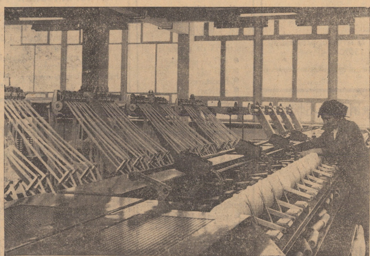
La unul din laminarele secției preparația filaturii de lînă pieptănată a fabricii „Liberfatea” Sibiu
