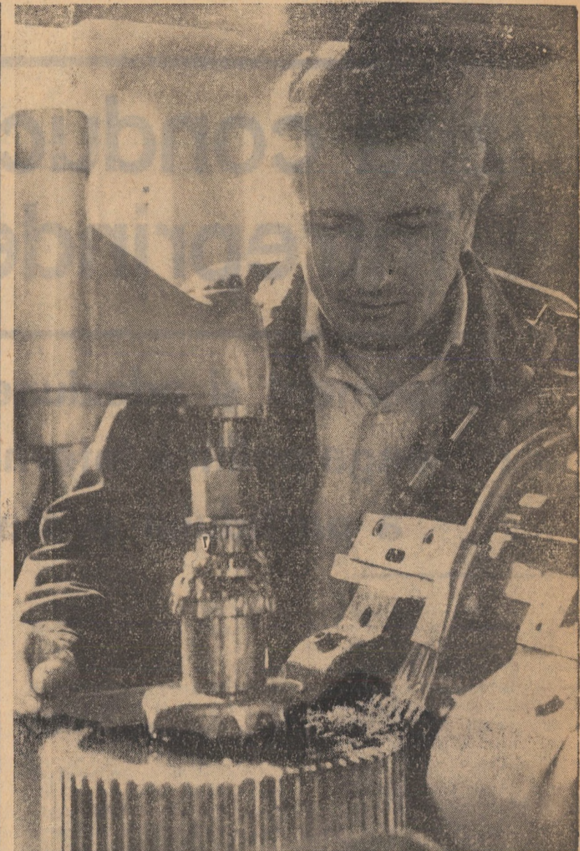
La o mașină de frezat prin rostogolire, frezorul Mircea Crăciun din atelierul secției mecanice al Uzinei „Independența” din Sibiu urmărește cu atenție prelucrarea unei roți dințate
