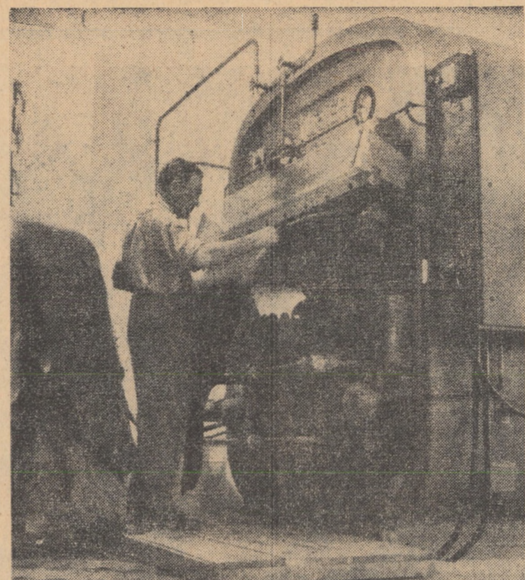
Un utilaj de mare productivitate la sectorul de tăbăcărie minerală al Fabricii de încălțăminte și piele — Agnita; presă pentru imprimarea feței pieilor finite. În 8 ore această mașină prelucrează 450 piei
